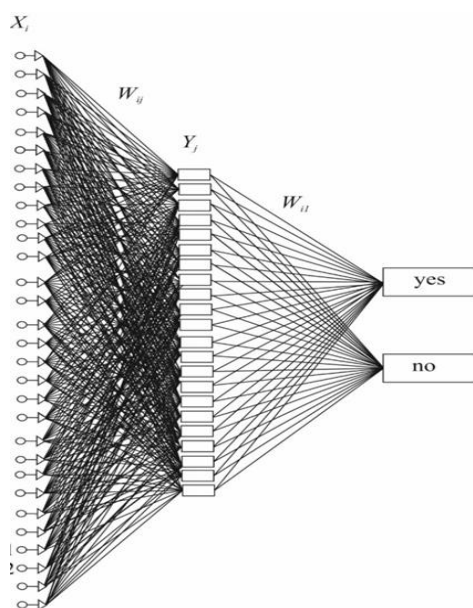
Рисунок 9 – Архитектура нейронной сети MLP 30-22-2
