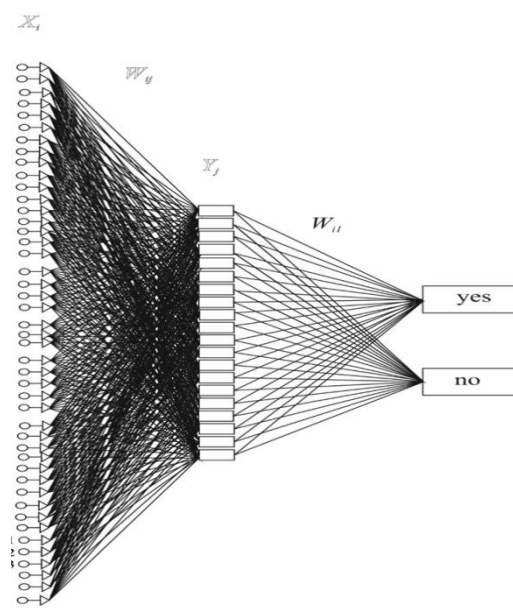
Рисунок 10 – Архитектура нейронной сети MLP 45-20-2
